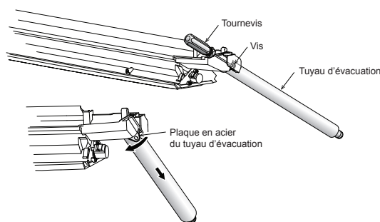
Tuyau d'évacuation
